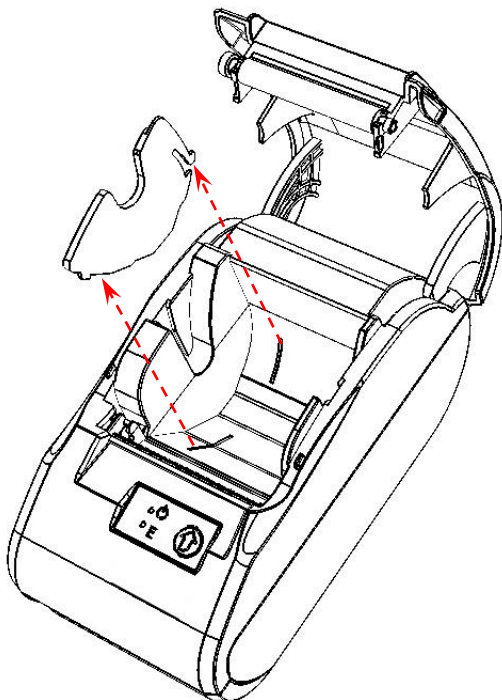
Рисунок 12. Извлечь ограничитель
